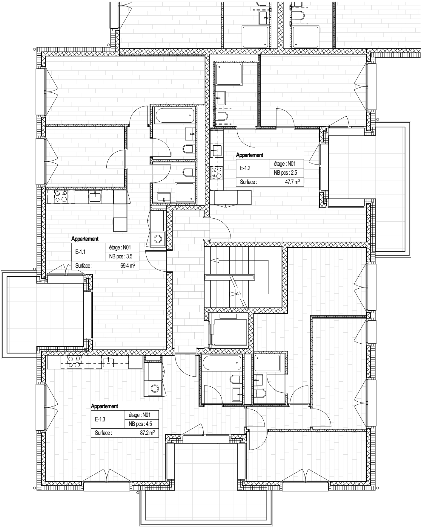
1 er étage
