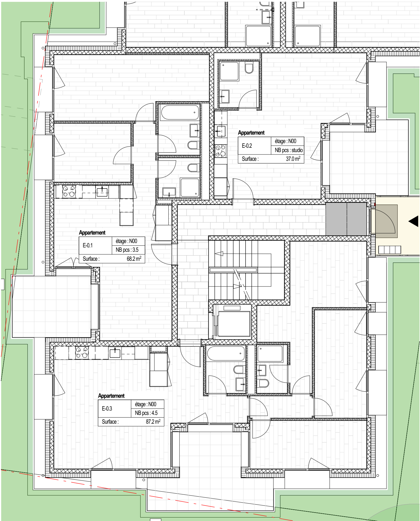
Rez-de-chaussée
