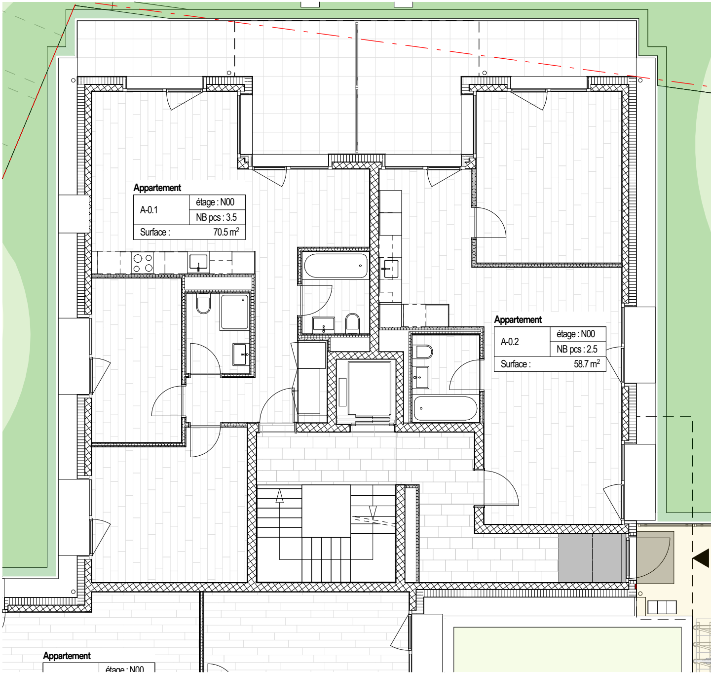
Rez-de-chaussée
